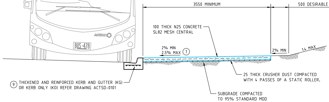
CROSS SECTION A-A N.T.S.
