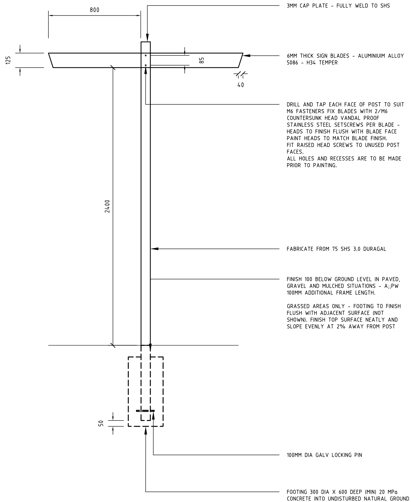
ELEVATION 1:20
