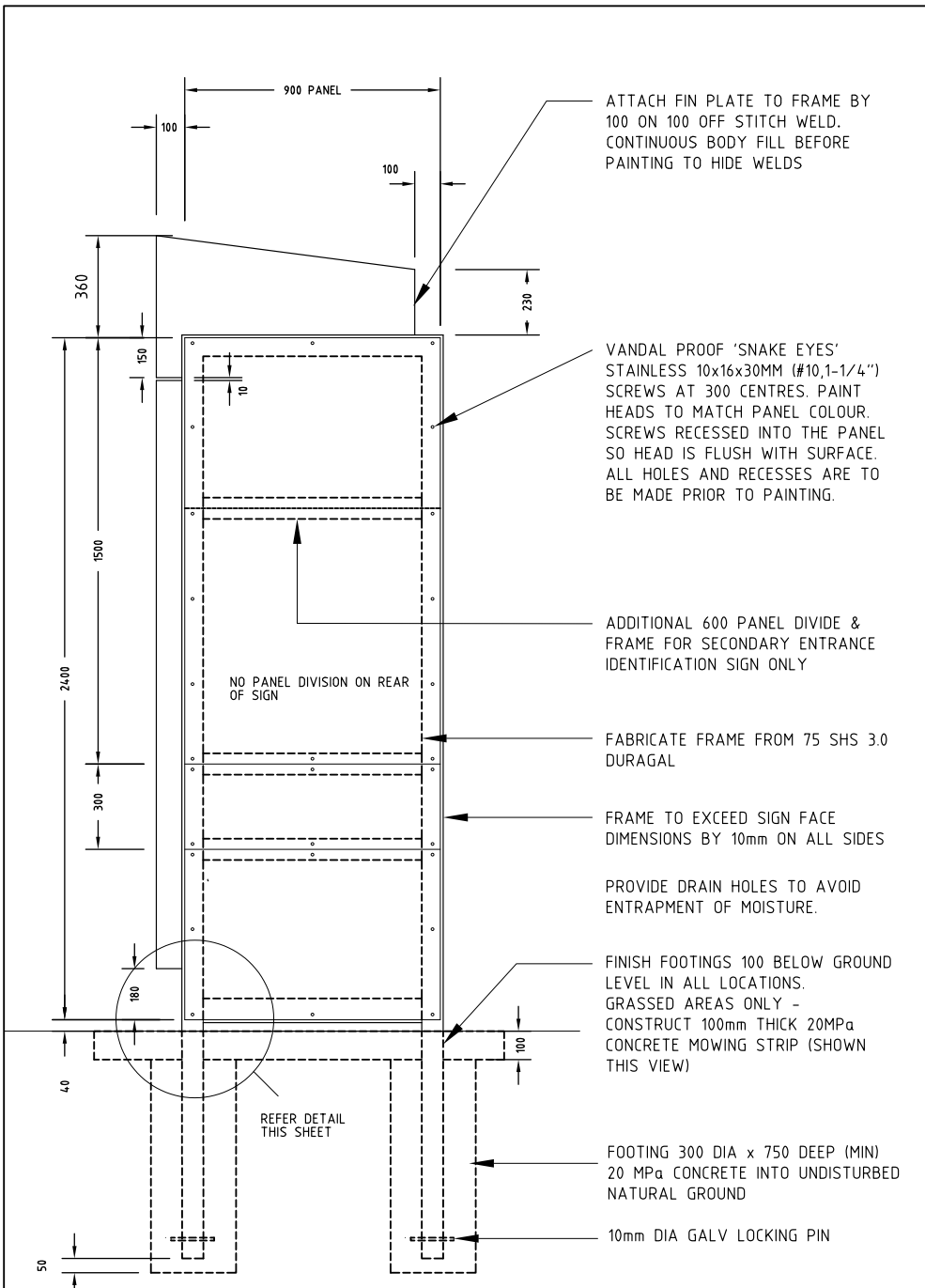
ELEVATION 1:25
